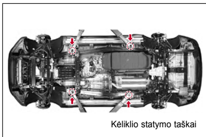
Automobilio kėliklio statymo taškas gale
